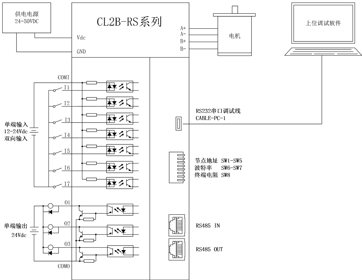
图 3-1 总线步进配线图
