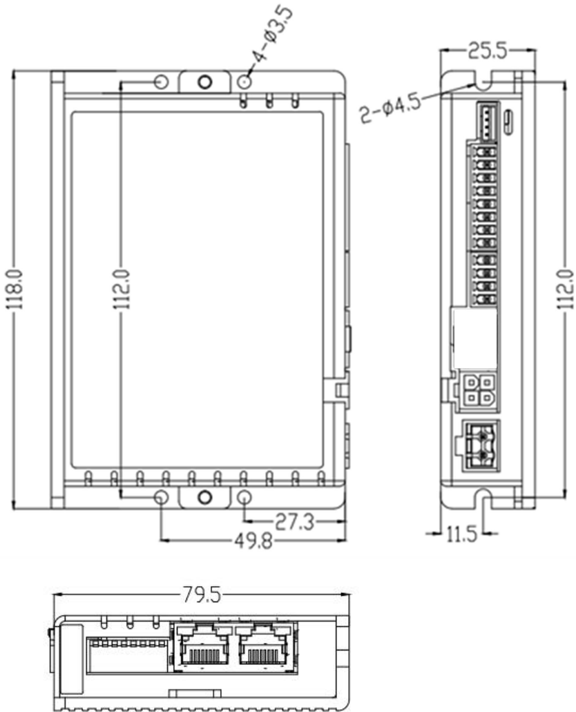
图 2-1 CL2B-RS503/507 系列驱动器机械尺寸
